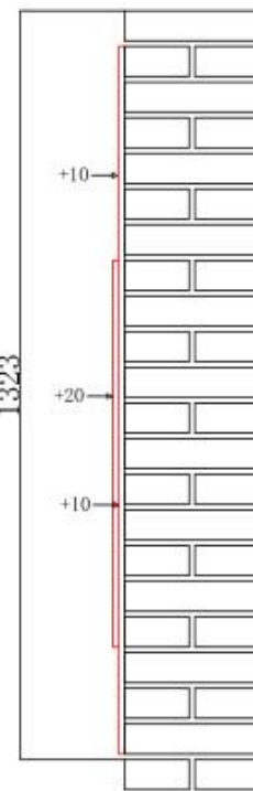
侧立面图
