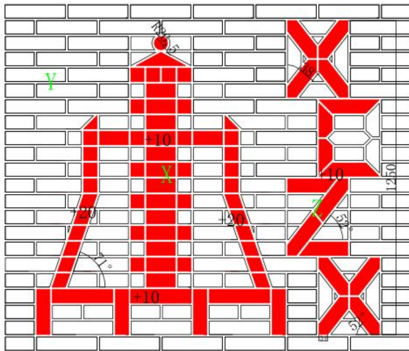
正立面图
